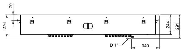
Boční
